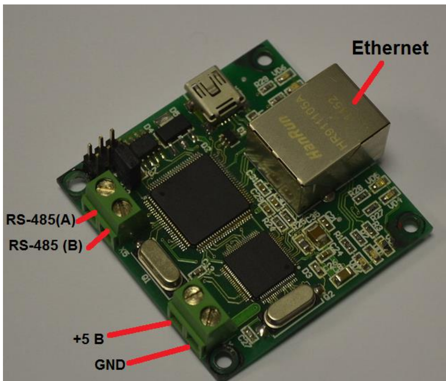
Рисунок 3.1 Внешний вид и обозначение соединителей конвертора Ethernet/RS-485 ТИШЖ.465449.103
